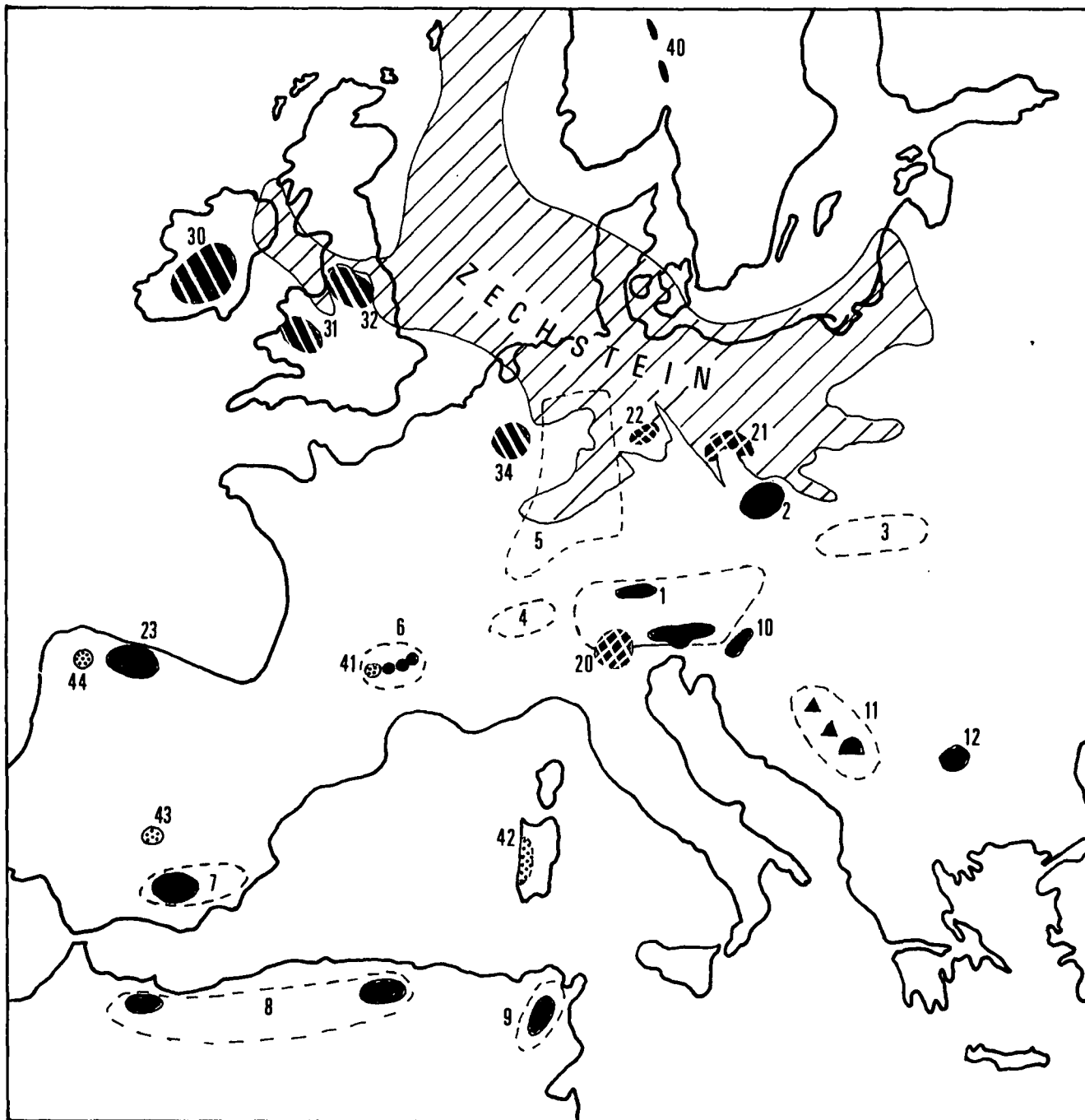
Abb. 5: Übersichtskarte an Karbonat- oder Sandsteinfazies schichtgebundener Pb-Zn-Lagerstätten Europas und des angrenzenden mediterranen Raumes (unter Verwendung von Daten von WOLF, 1981; FONTBOTÉ & AMSTUTZ, 1983 u. a.).
